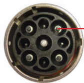
JUICE CONNECTOR 上の 感電防止タッチガード (m)
