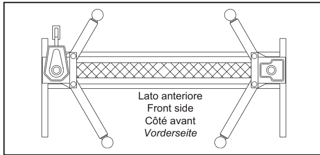
Fig.40 Disposizione dei bracci
