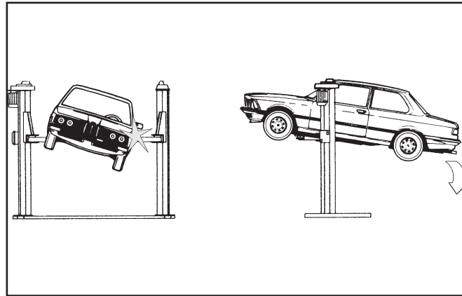
Fig.14 - Abb.14 Rischio di caduta del veicolo Risk of vehicle fall Risque de chute du véhicule Absturzgefahr des Fahrzeugs Peligro de caída del vehículo
